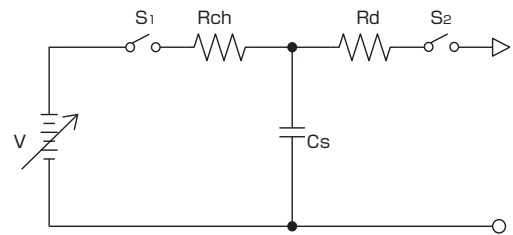
コンデンサ容量 Cs:150pF 放電抵抗 Rd:330Ω
