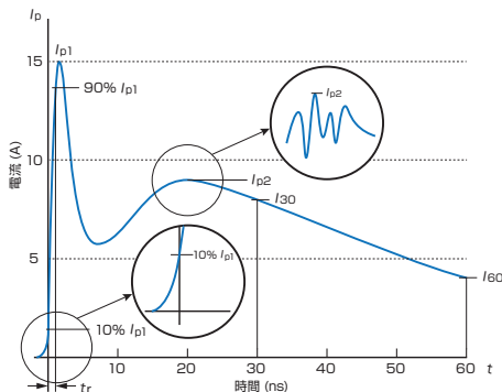
4kVにおける接触放電の放電電流波形
