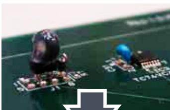
フェライトコアによる対策
