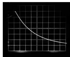
電圧サージ波形：1.2/50 \mu s 電圧：3kV V：500V/Div H：20 \mu s /Div
