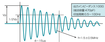
<インパルス波形(方形波)>
