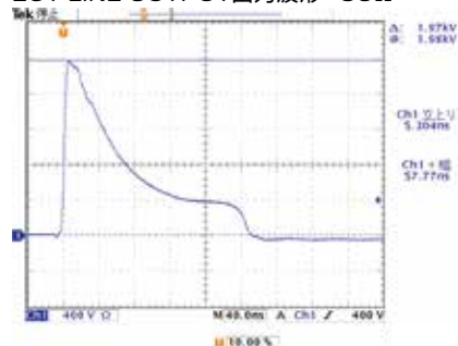
EUT LINE OUTPUT出力波形：50Ω
