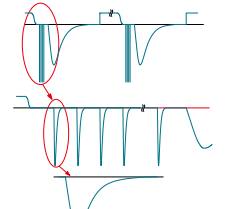
<フィールドディケイノイズ+火花サージ(バースト波形)>
