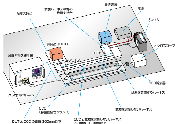
ISO 7637-3【容量性結合クランプ法 (CCC 法)】
