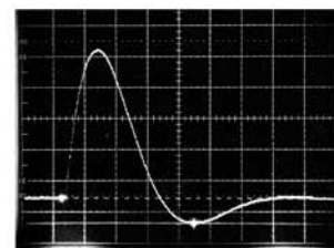
電流サージ波形：8/20 \mu s 電流：2400A I：500A/Div H：10 \mu s /Div
