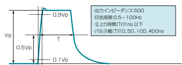
<インパルス波形(方形波)>
