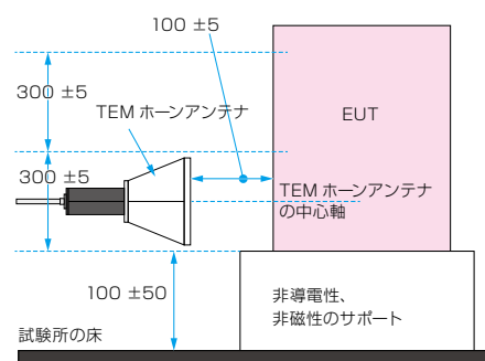
TEMホーンアンテナを使用した床置き型EUTへの試験イメージ (380 MHz ~ 6 GHz)
