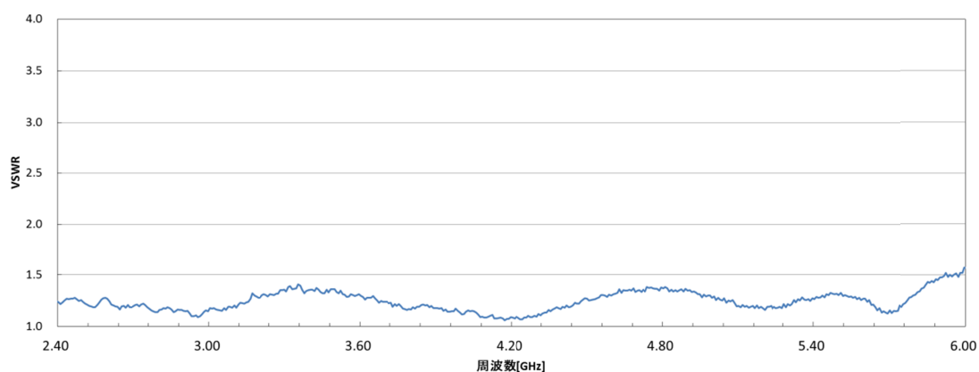
VSWR 参考特性
