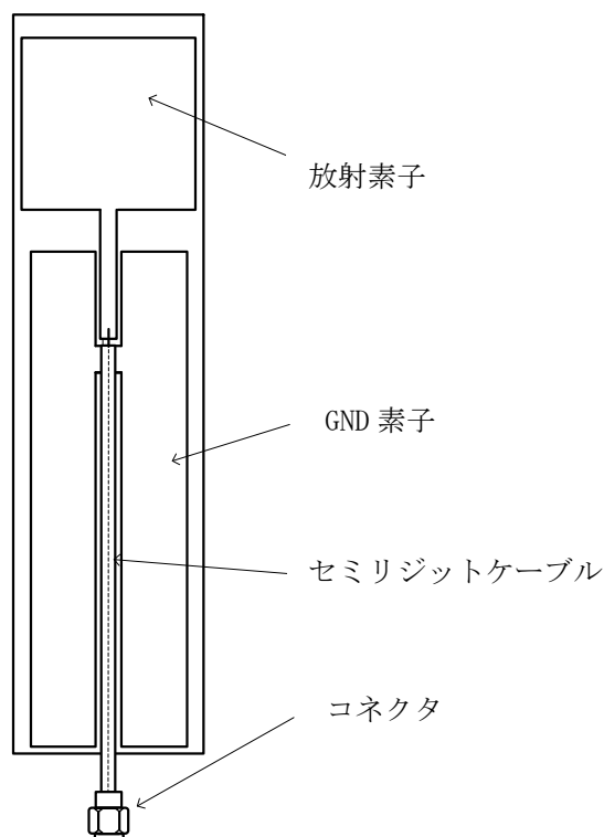
NKU2460G のアンテナパターン(イメージ)
