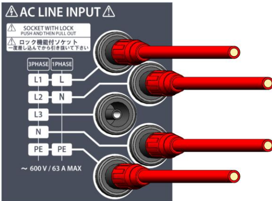
単相三線 PE ありの場合
