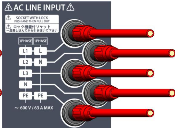
三相四線 PE ラインあり
