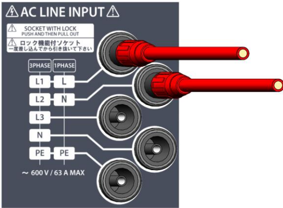
PE ラインなしの場合
