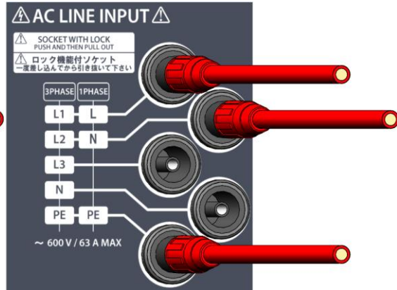
PE ラインありの場合
