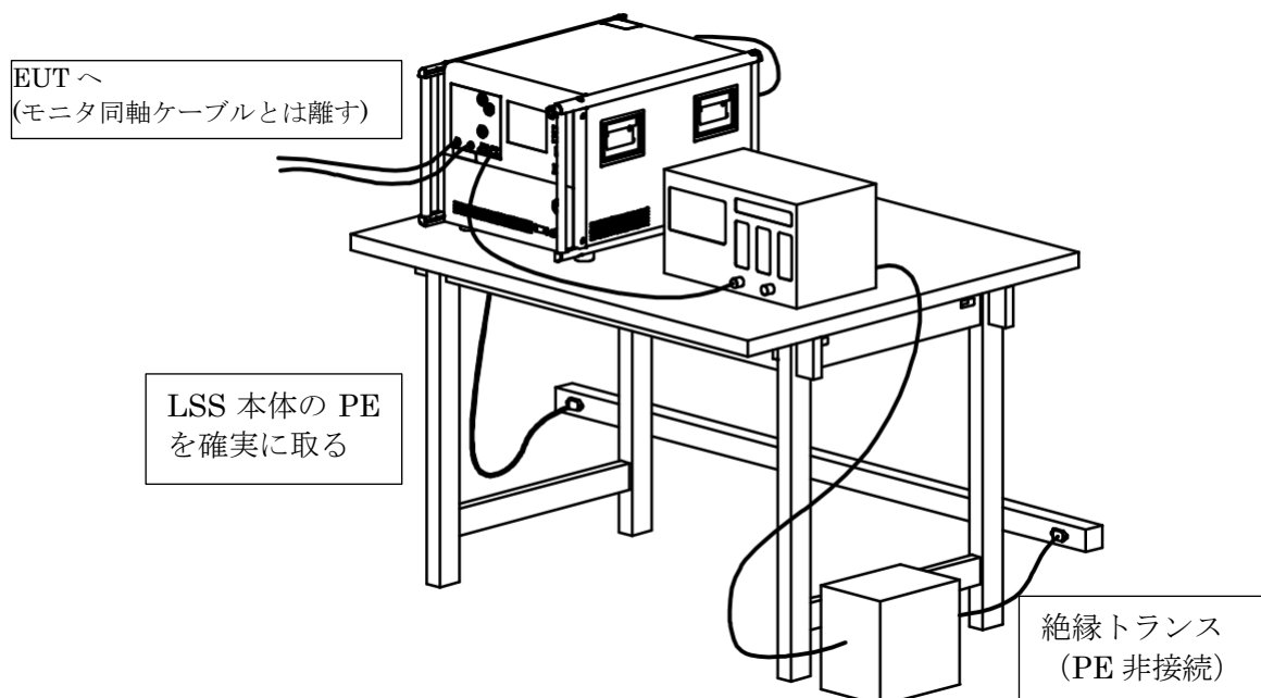
図 21-1. モニタ測定時の接続
