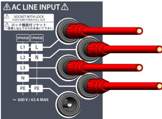
三相四線 PE ラインなし
