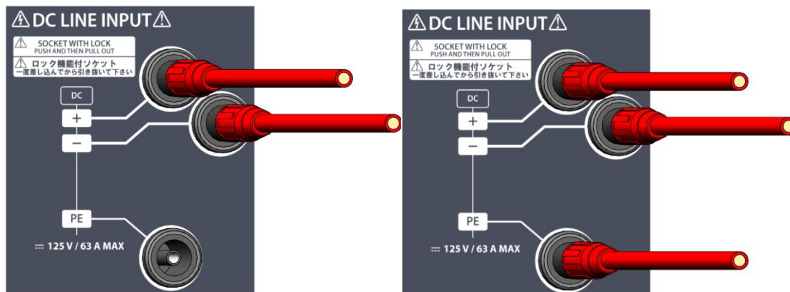
PE ラインなしの場合
