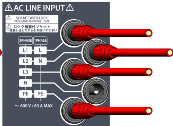
三相三線 PE ラインあり
