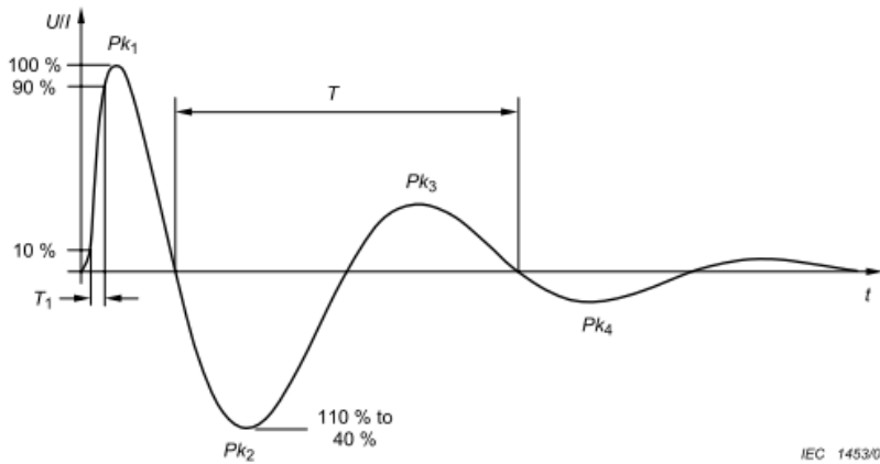
図 8-2 RINGWAVE 電圧サージ波形
