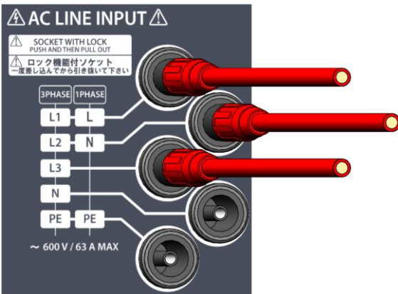
三相三線 PE ラインなし
